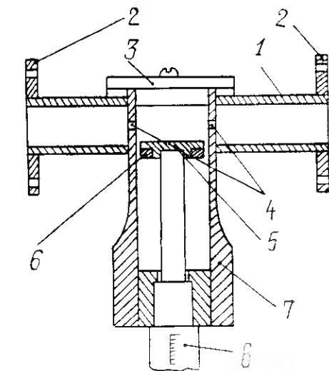
Рис. 15. Конструкция волномера с цилиндрическим резонатором на волну H_{01n} . 1. Волновод. 2. Контактные фланцы. 3. Крышка. 4. Диафрагмы связи. 5. Поршень. 6. Кольцо для подавления нежелательных типов волн. 7. Цилиндр. 8. Микрометрическая головка.
