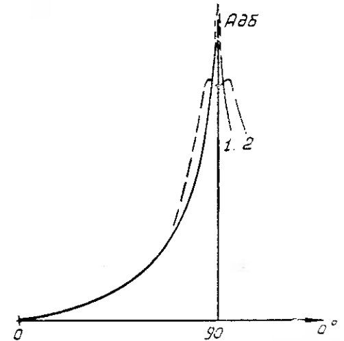
Рис. 60. Искажения градуировочной кривой поляризационного ослабителя. 1. Идеальная кривая. 2. Реальная кривая.
