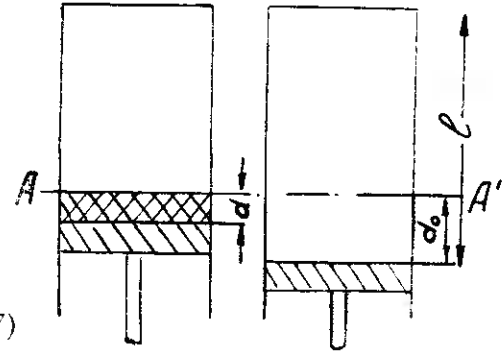
Рис. 77. Схема объемного резонатора с образцом диэлектрика и без образца.
