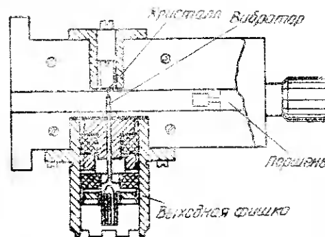
Рис. 6. Конструкция детекторной головки миллиметрового диапазона.
