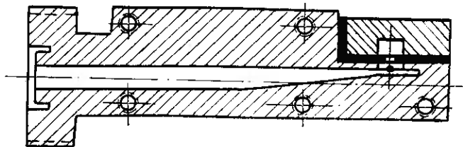
Рис. 34. Схема ненастраиваемой термисторной головки.
