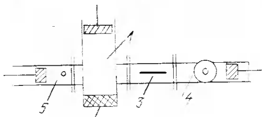
Рис. 78. Схема установки для измерения диэлектриков резонаторным методом.
