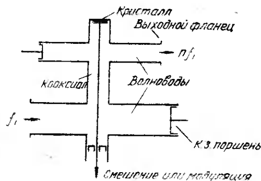
Рис. 3. Принципиальная схема умножения частоты с помощью кристаллического детектора.
