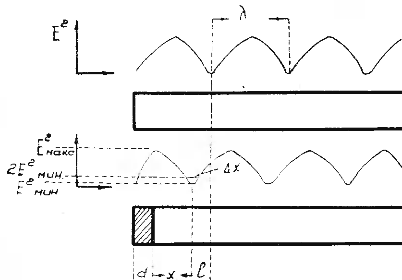
Рис. 72. Распределение поля в короткозамкнутом волноводе без образца и с образцом диэлектрика.
