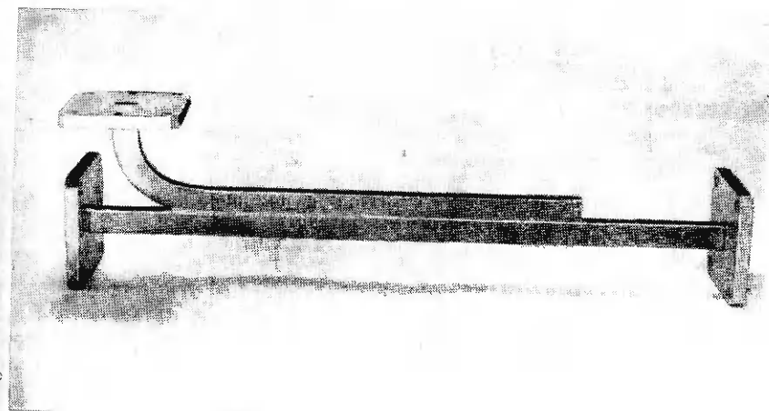
Рис. 65. Внешний вид направленного ответвителя с элементом связи в виде решетки.
