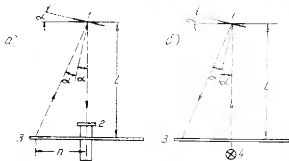
Рис. 51. Индикаторные устройства: а) с зрительной трубой, б) со шкалой.
