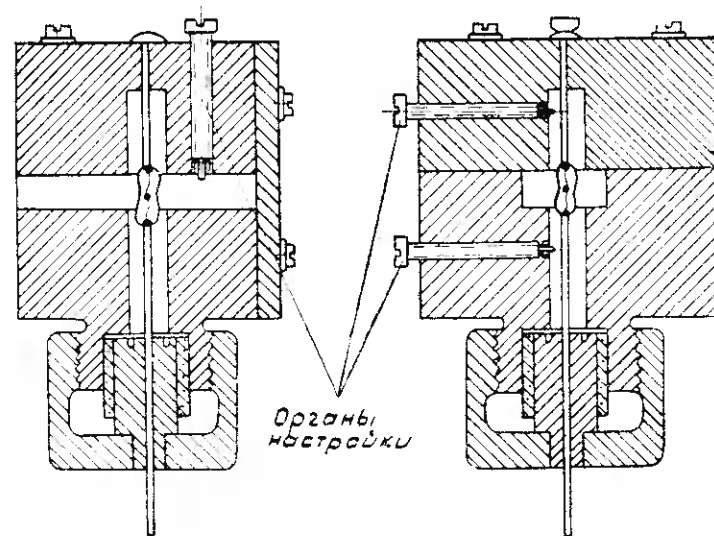
Рис. 33. Конструкция настраиваемой термисторной головки.
