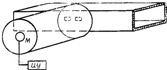
Рис. 40. Мембрана в стенке объемного резонатора, присоединенного к волноводу.
