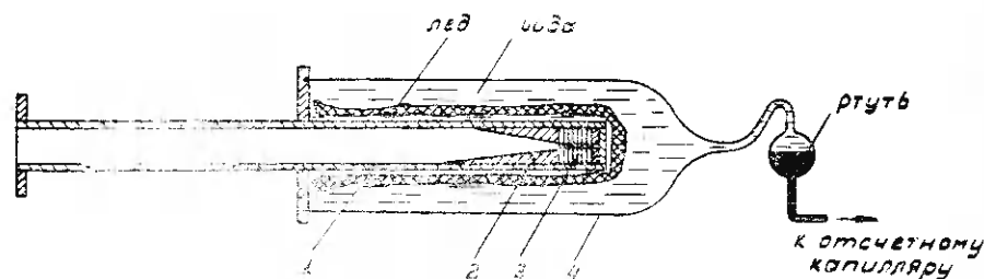
Рис. 30. Схема ледяного калориметра.
