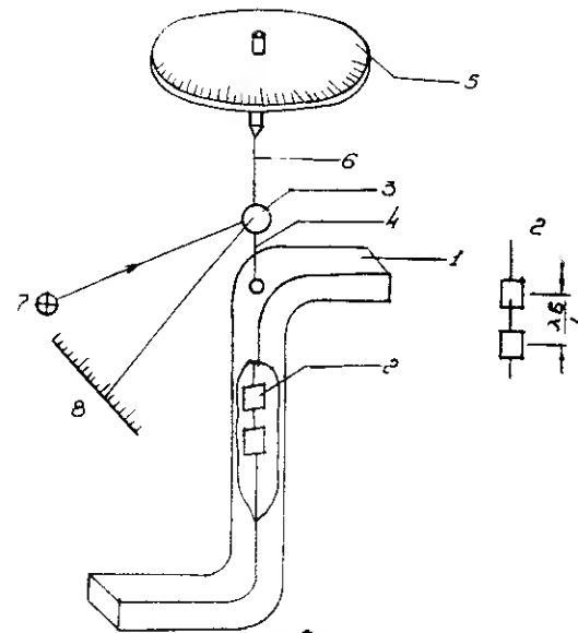
Рис. 56. Схема пондеромоторного ваттметра с двумя чувствительными элементами.
