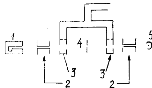
Рис. 19. Принципиальная схема цезиевого эталона частоты.
