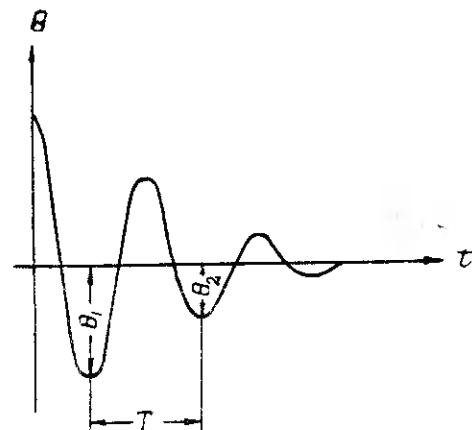
Рис. 53. График колебаний при механической градуировке чувствительного элемента пондеромоторного измерителя мощности.
