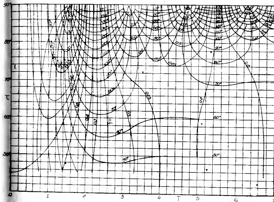
Рис. 73. График функции \frac{th Te^{i\tau}}{Te^{i\tau}} = Ce^{i\xi} .
