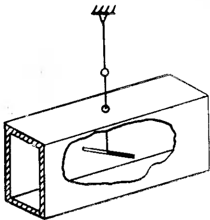
Рис. 46. Схема пондеромоторного измерения мощности с несимметричным чувствительным элементом.
