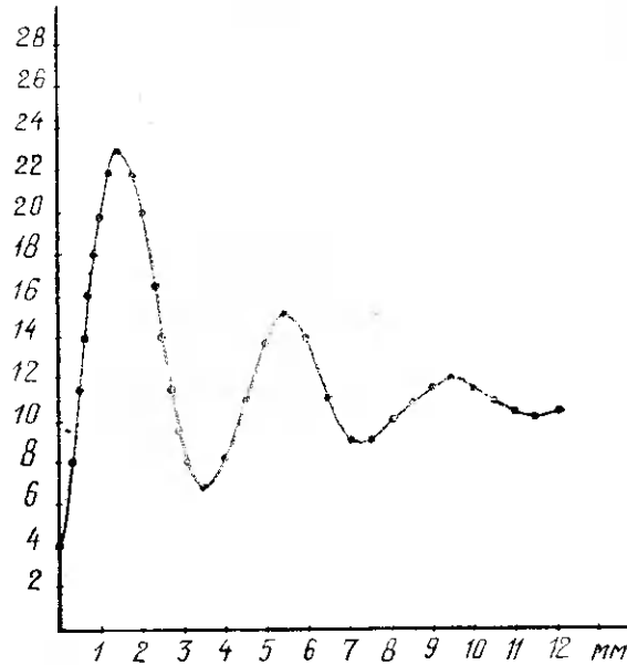
Рис. 76. График затухания электромагнитных волн в жидком диэлектрике.
