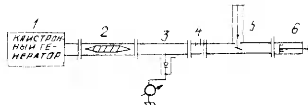
Рис. 54. Блок-схема при градуировке пондеромоторного измерителя мощности.
