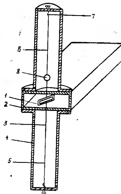
Рис. 49. Схема пондеромоторного ваттметра для относительных измерений мощности.
