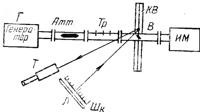
Рис. 86. Блок-схема установки для измерения диэлектриков с помощью пондеромоторного измерителя.
