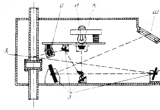
Рис. 52. Конструкция индикаторного устройства для переносного пондеромоторного измерителя мощности.
