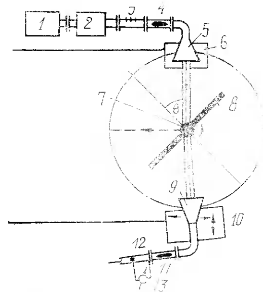
Рис. 85. Блок-схема установки для измерения диэлектриков в свободном пространстве. 1 — Генератор. 2 — Волномер. 3 — Трансформатор. 4 — Аттенюатор. 5 — Передатчик. 6 — Механическое устройство для перемещения передатчика. 7 — Механическое устройство для перемещения образца испытуемого материала. 8 — Испытуемый образец. 9 — Приемный рупор. 10 — Приемник. 11 — Индикатор. 12 — Механическое устройство для перемещения приемной антенны.
