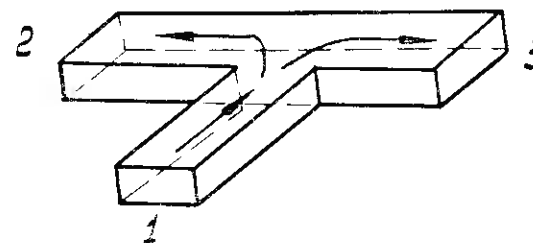
Рис. 68. Схема устройства волноводного тройника.
