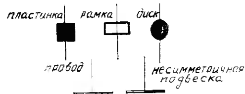
Рис. 50. Чувствительные элементы для пондеромоторных измерителей мощности.
