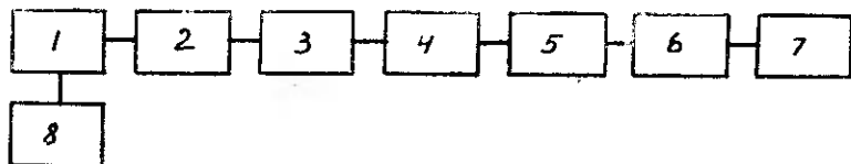
Рис. 71. Блок-схема для градуировки ослабителей методом квадратичного детектора.
